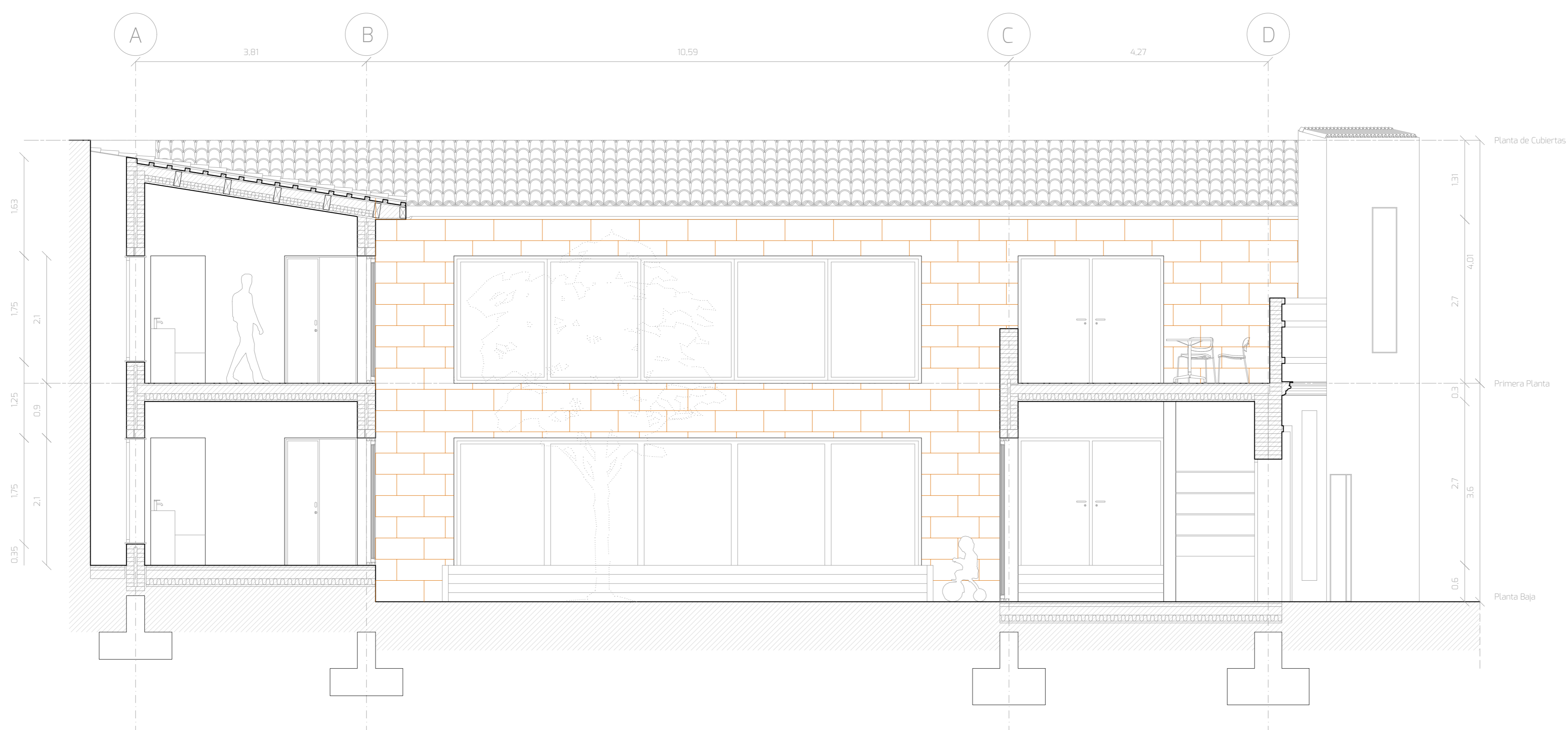
sección d-d'
