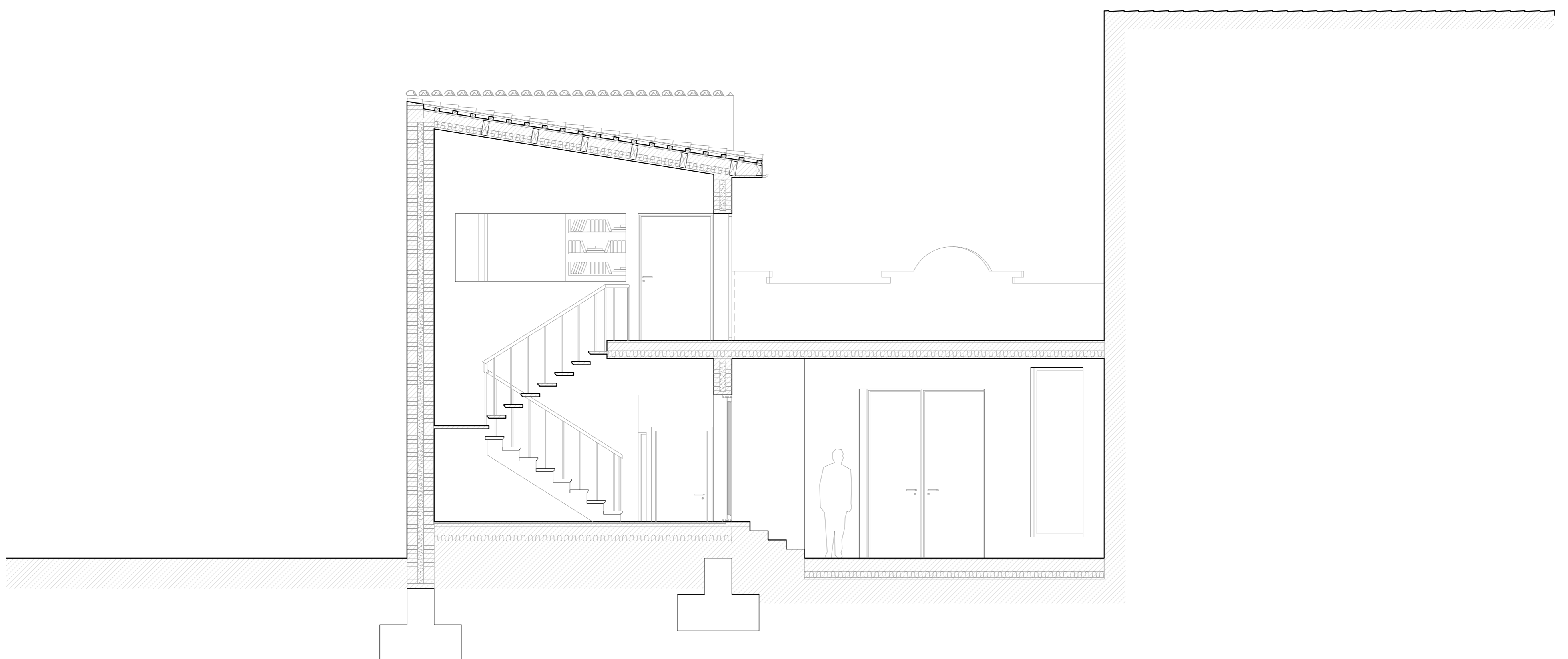
sección c-c'
